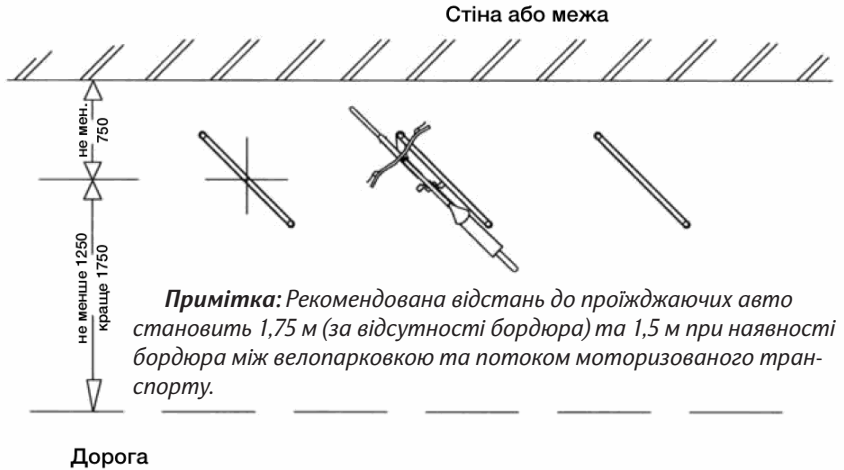
Мал. 4: П-подібні стійки, розташовані під кутом 45 градусів до стіни та потоку моторизованого транспорту
