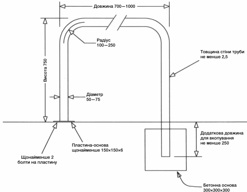
Мал. 1: Базова П-подібна стійка
